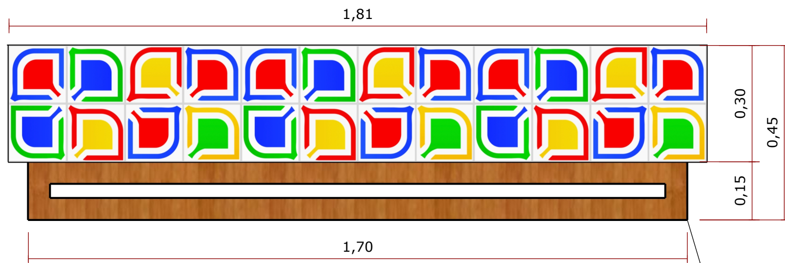
BANCO REVESTIDO COM AZULEJOS PERSONALIZADOS COM A LOGO DA AGÊNCIA
