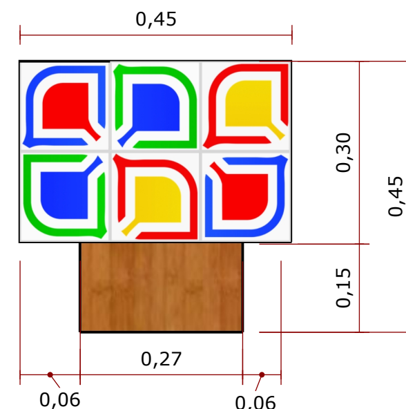
VISTA LATERAL DO BANCO
